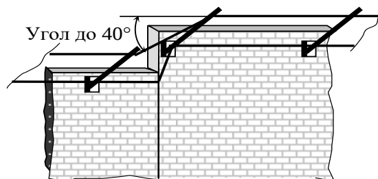
Рисунок 2.3 – Крепление КМЧ и проводов при перепадах высоты
